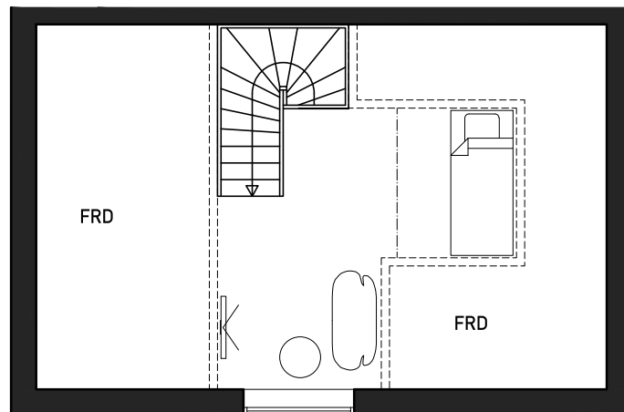
HUS 1D VIND
